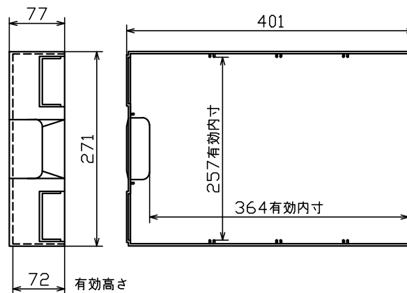
引出詳細図
