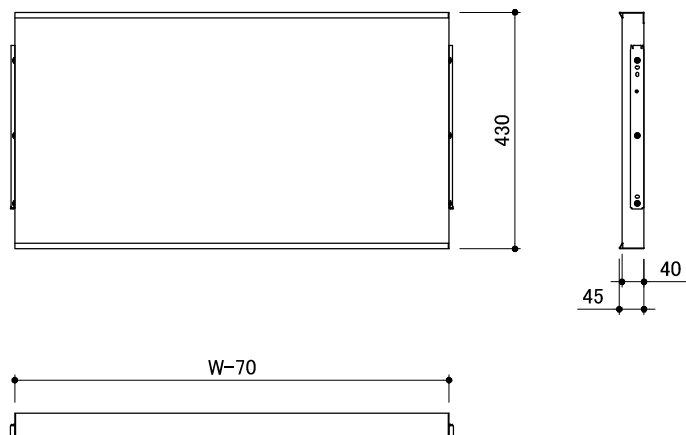
M1.5、M2型棚板 D445(450)用
