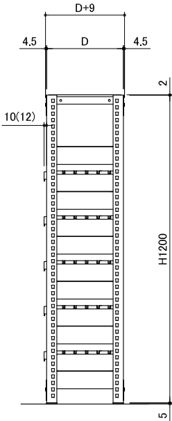
側面図
