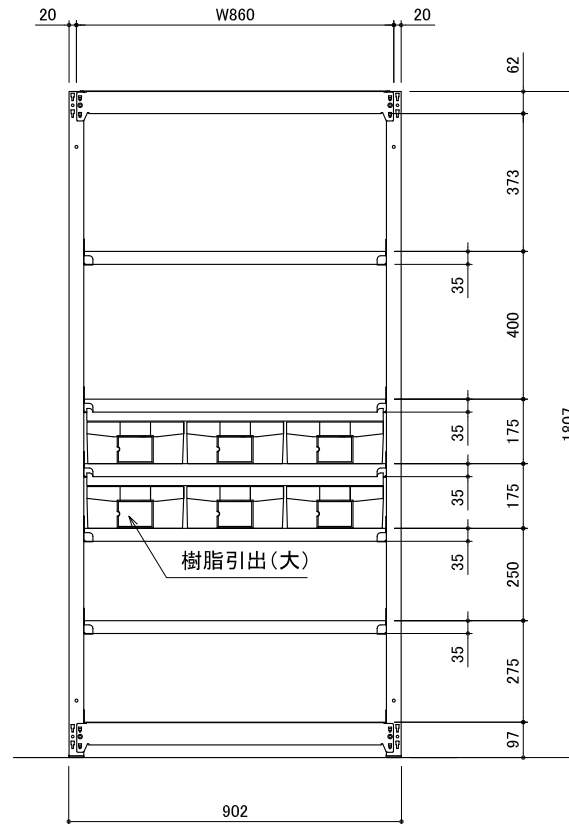
立面図 樹脂引出(大)6個
