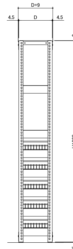
側面図
