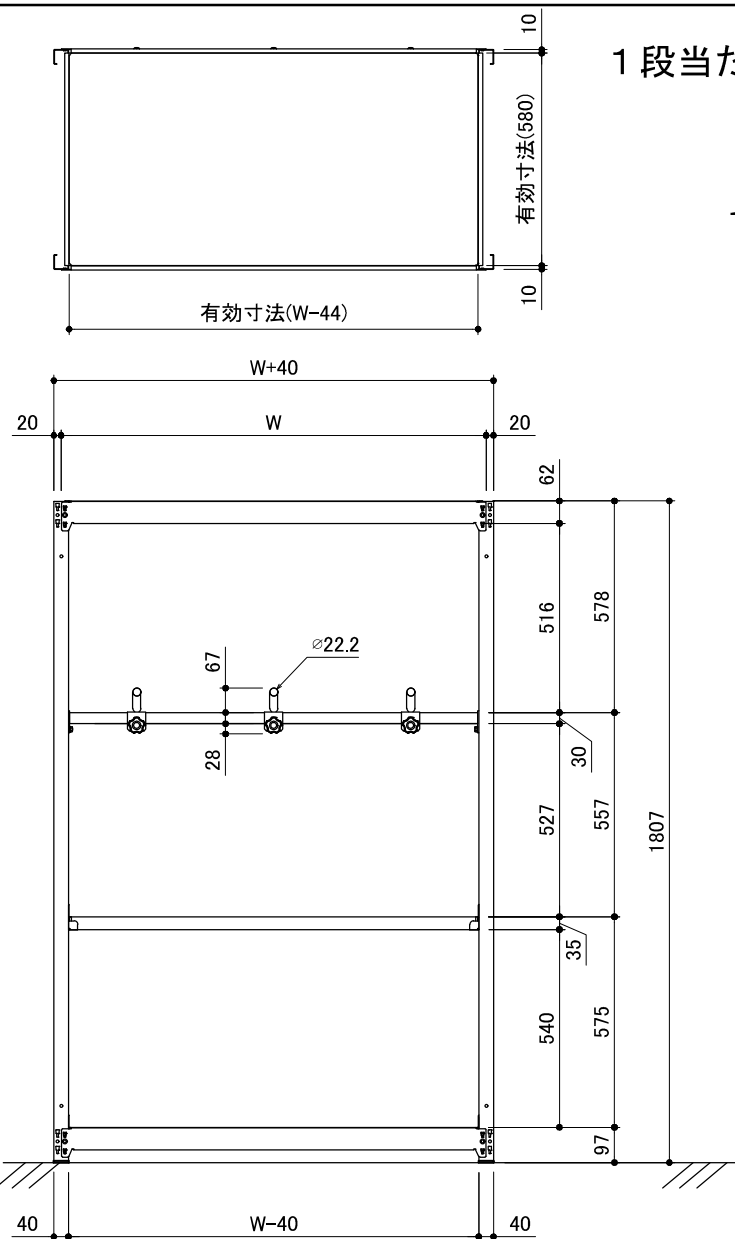
単体型
