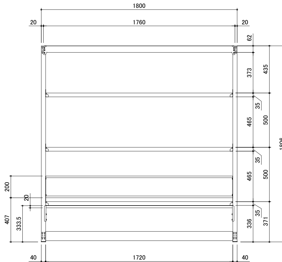
単体型
