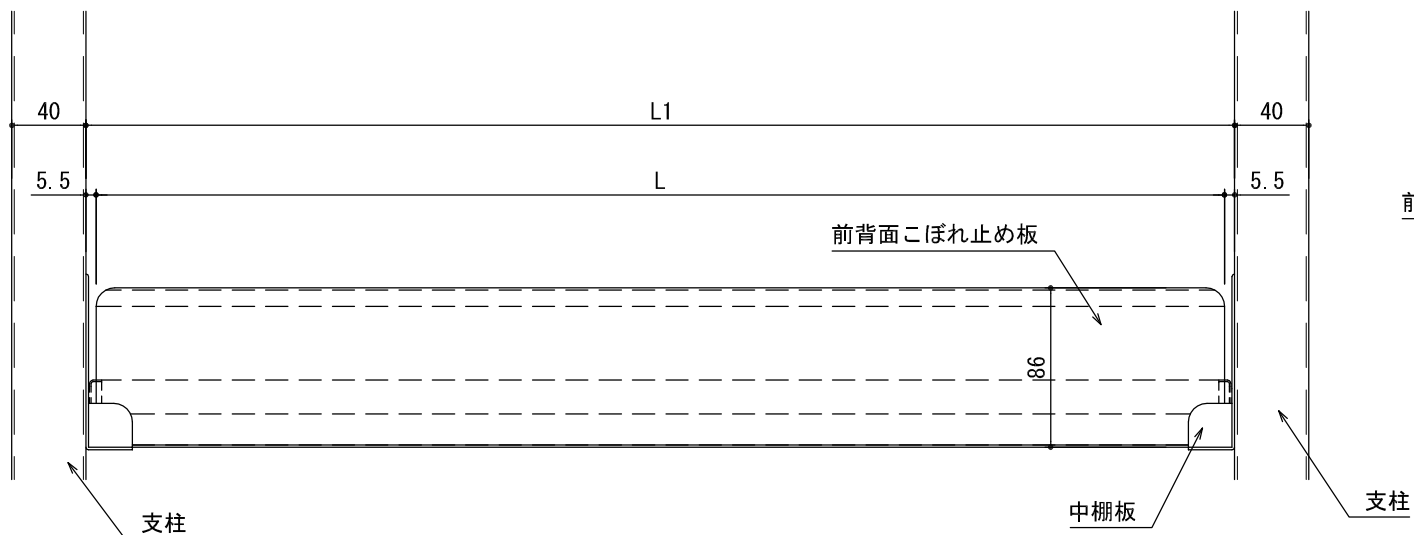
取付図 (M2型)
