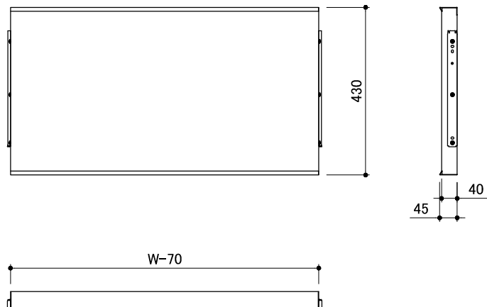
M1.5、M2型棚板 D445(450)用
