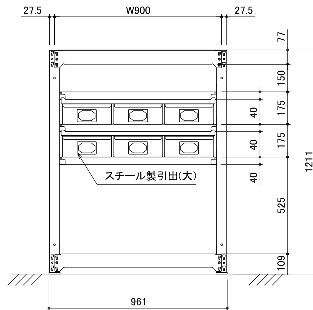
立面図 スチール製引出(大)6個
