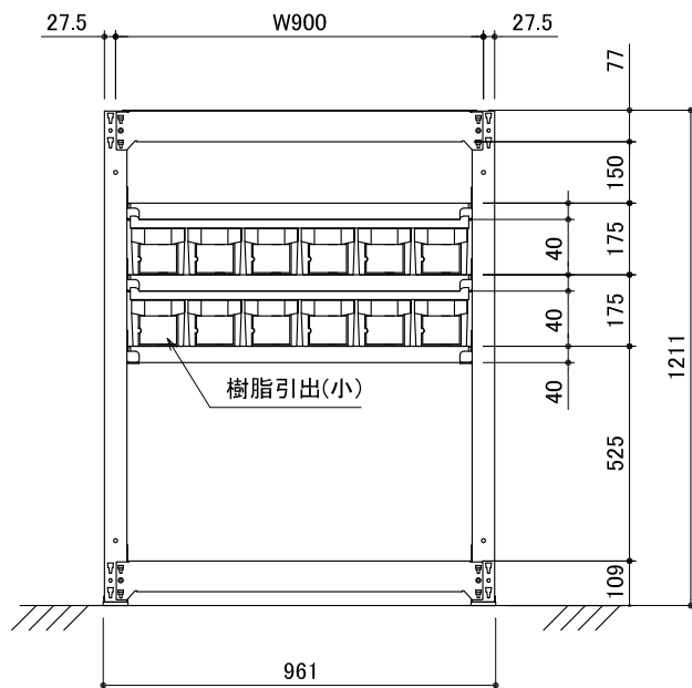
立面図 樹脂引出(小)12個
