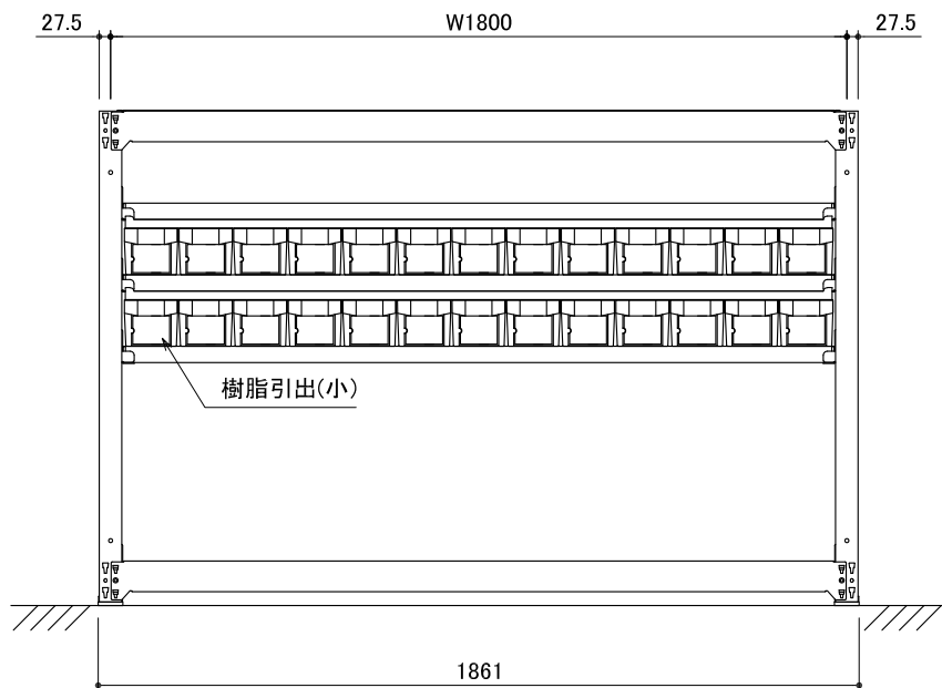
立面図 樹脂引出(小)26個
