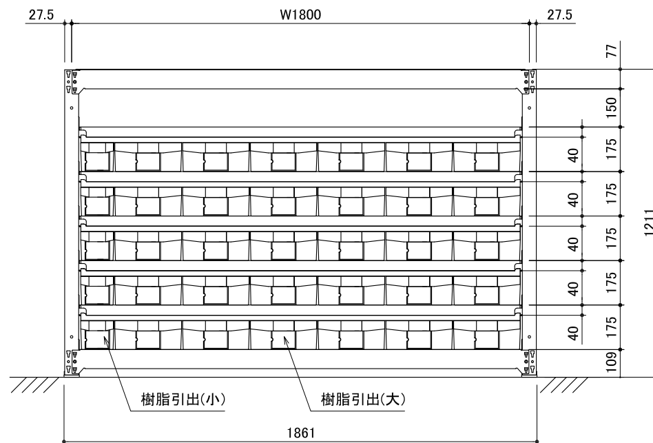
立面図 樹脂引出(大)30個、(小)5個
