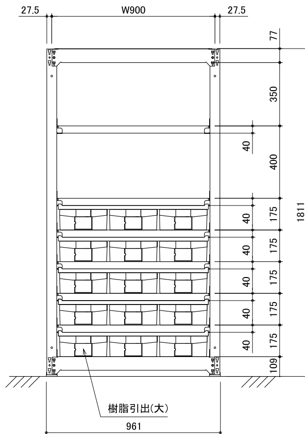
立面図 樹脂引出(大)15個
