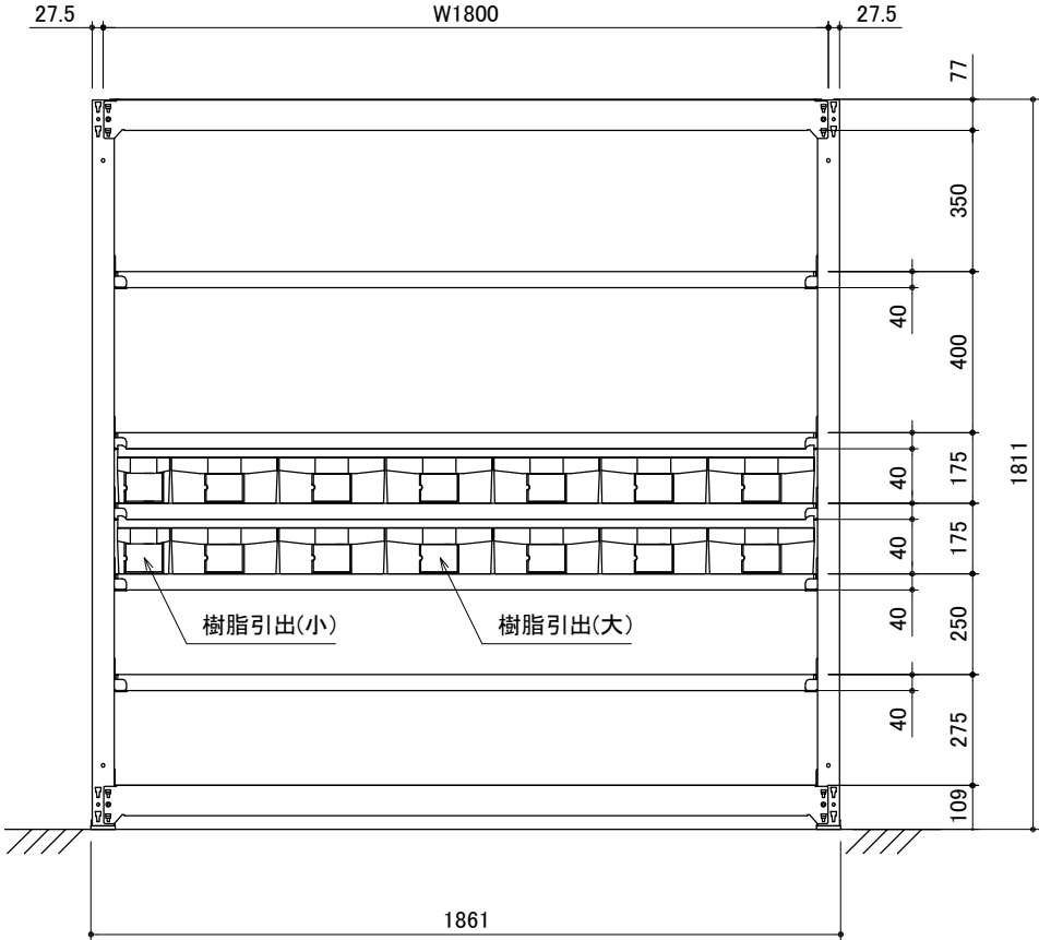
立面図 樹脂引出(大)12個,(小)2個
