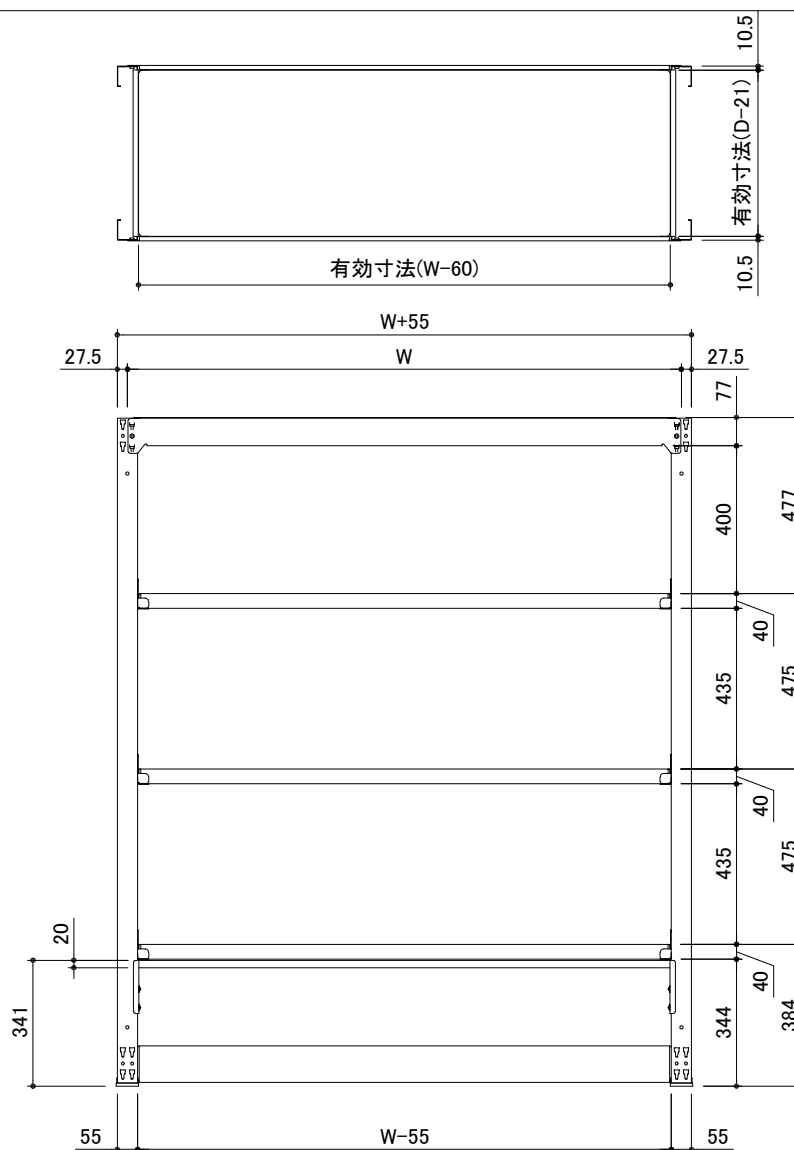
単体型
