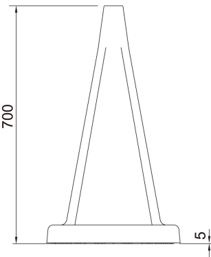
正面图(A面)
