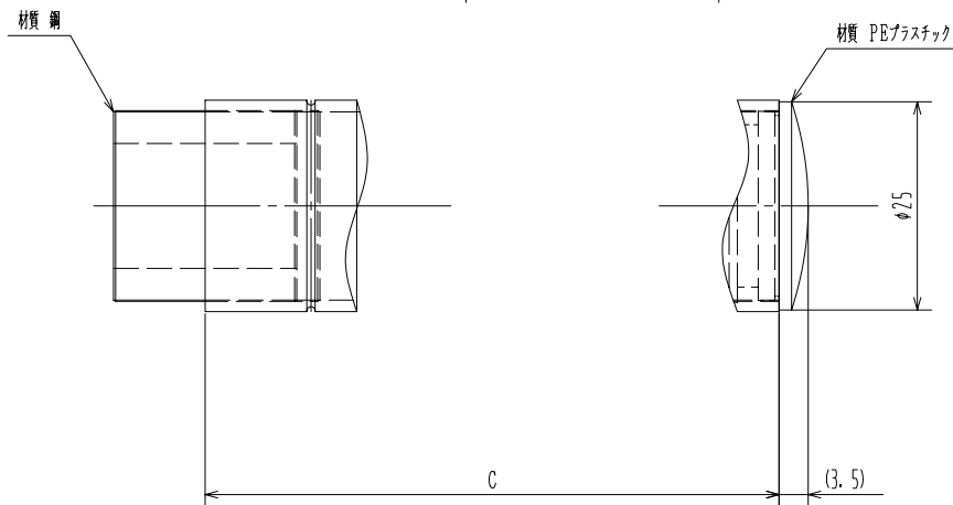
ねじ、キャップ取付詳細
