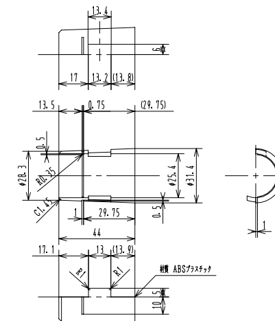
付属品 スリーブ詳細
