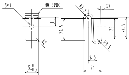
付属品 棚用連結金具詳細
