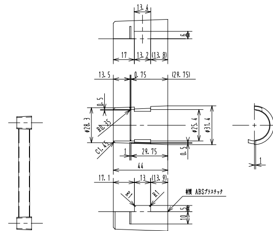
付属品 スリーブ詳細
