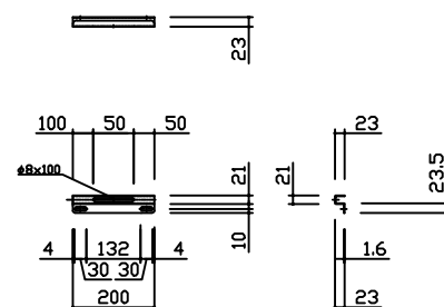
傾斜棚受け B
