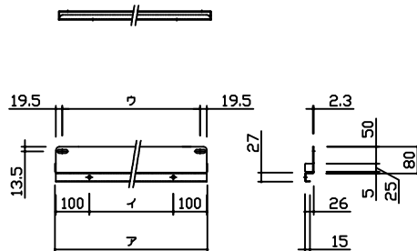
傾斜棚受け A
