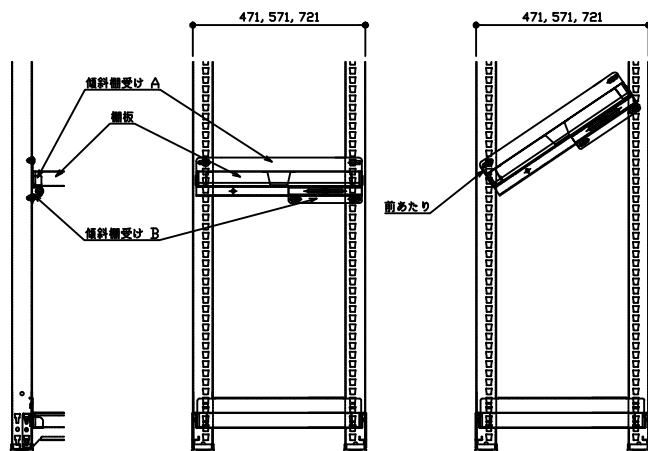
傾斜棚使用状態
