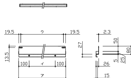
傾斜棚受け A
