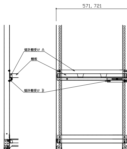
傾斜棚使用状態
