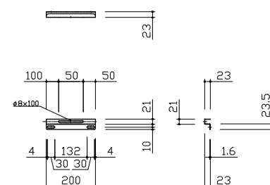
傾斜棚受け B
