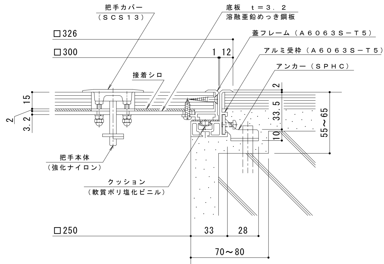
断面詳細図 S = 1 : 2
