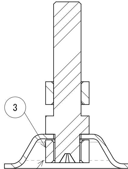
断面図 A-A ナット圧入
