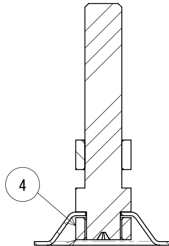
断面図 A-A
