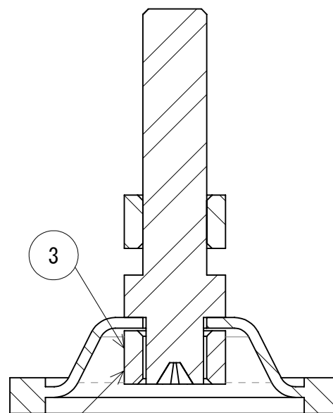
断面図 A-A
