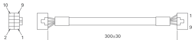
コネクタ間結線
