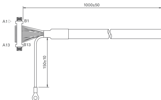
CN配線
