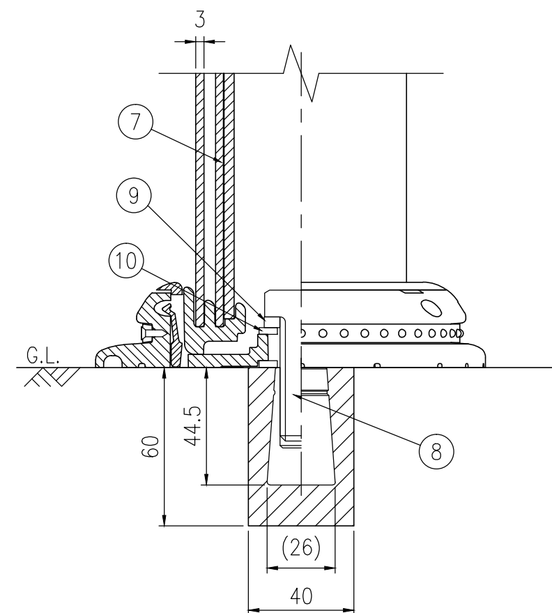
A-A半断面図 S=1/2
