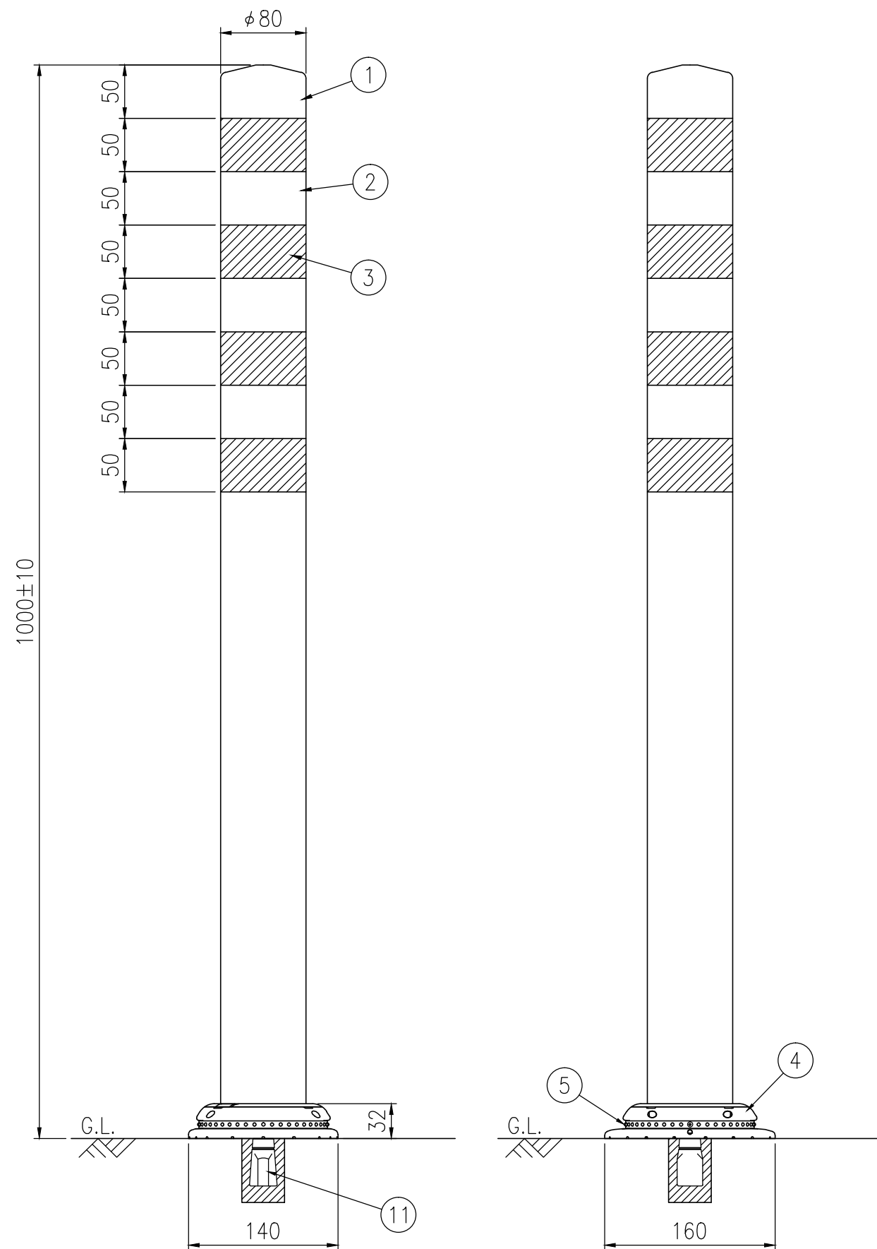
設置図 S=1/5
