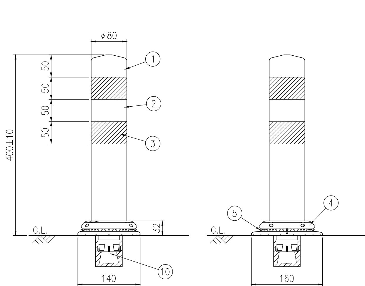
設置図 S=1/5
