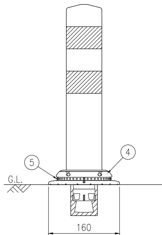
設置図 S=1/5
