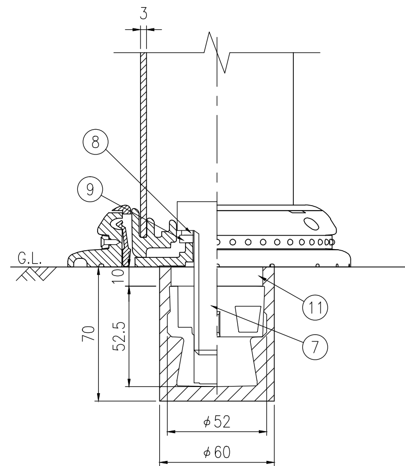
A-A半断面図 S=1/2
