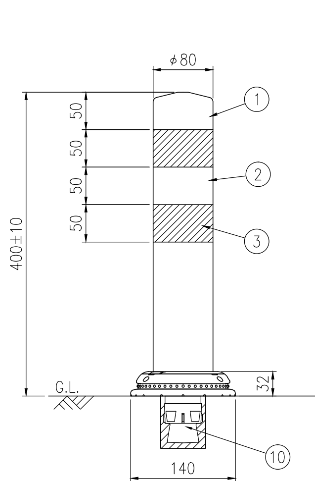
設置図 S=1/5
