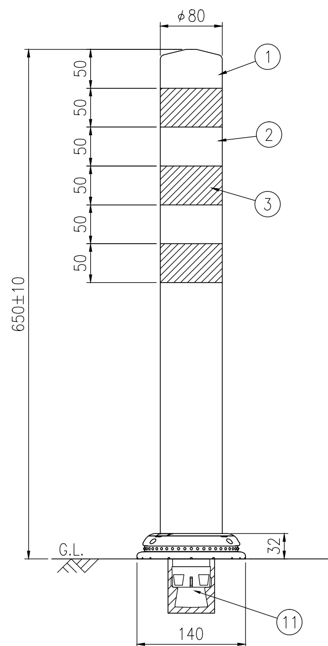
設置図 S=1/5
