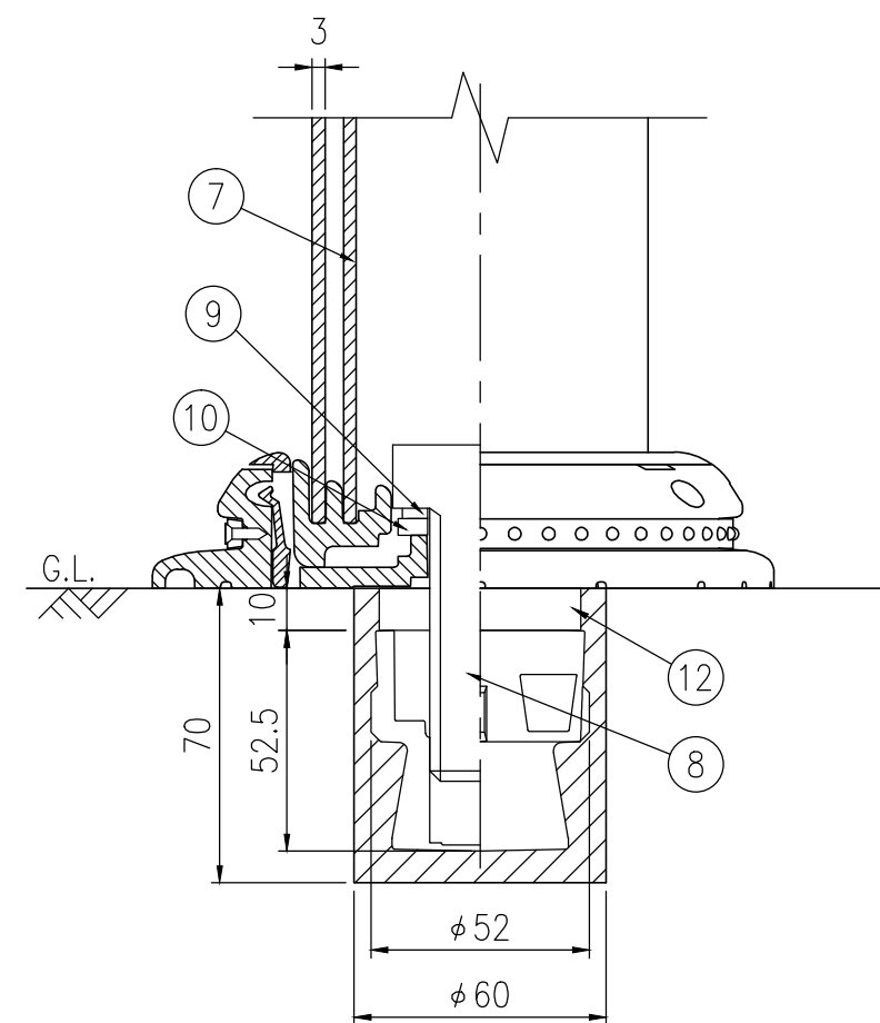
A-A半断面図 S=1/2
