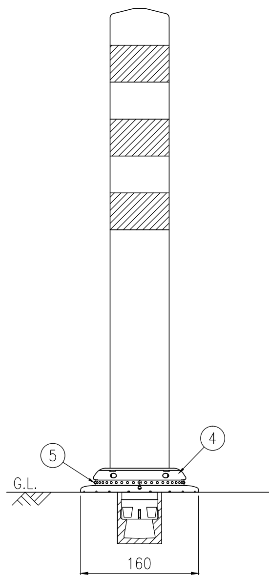
設置図 S=1/5
