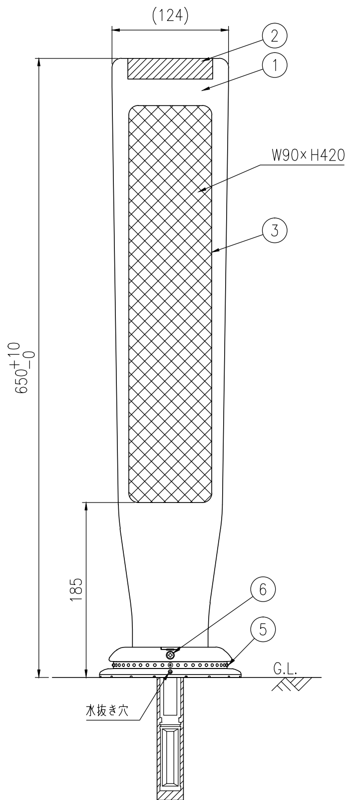
設置図 S=1/4
