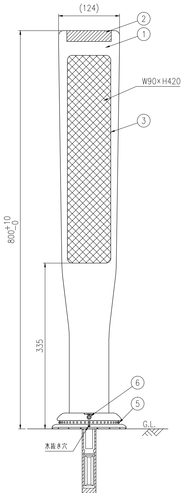
設置図 S=1/4
