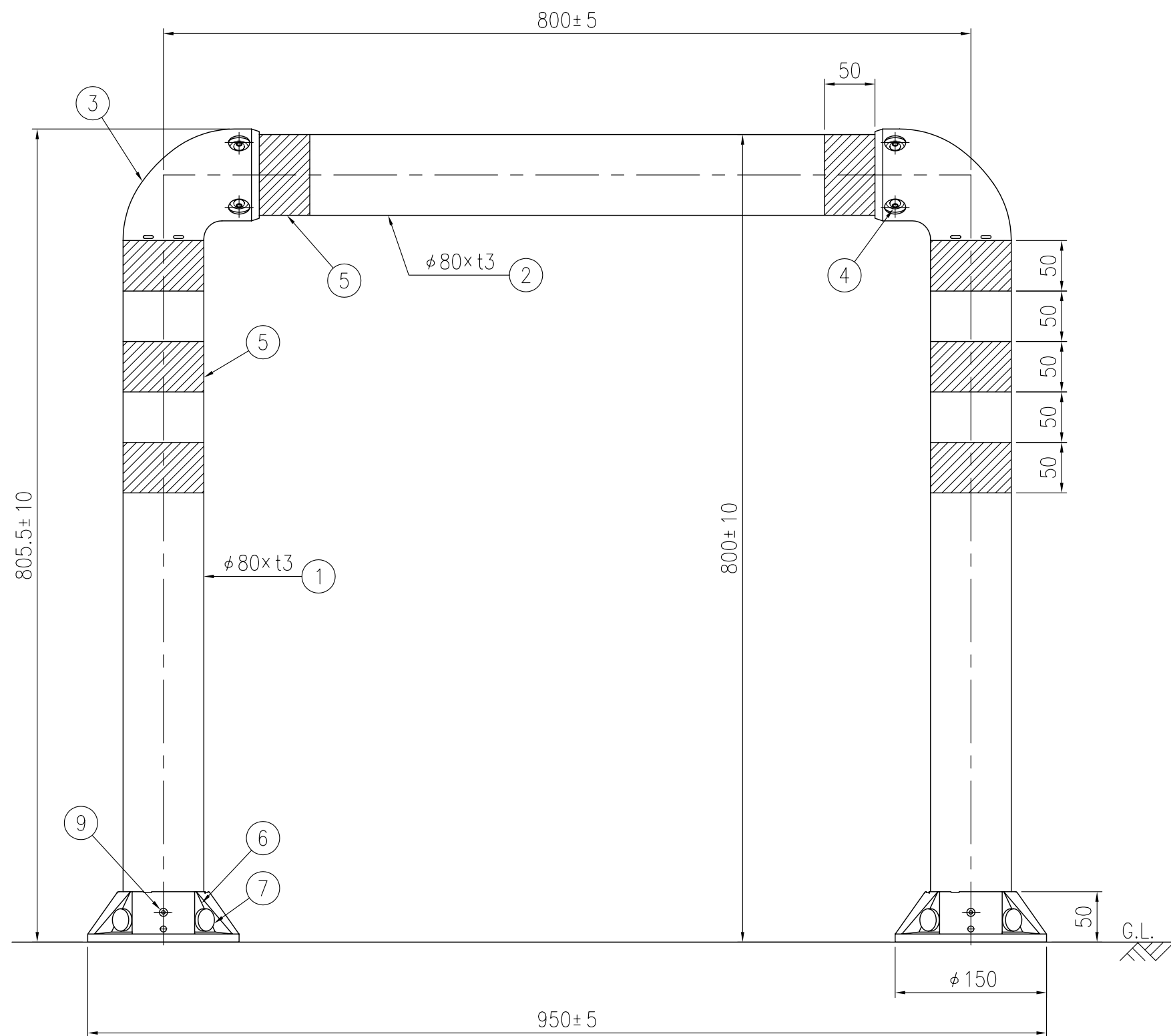
設置図 S=1/5
