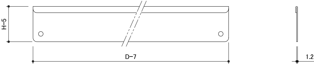
仕切(平行用)
