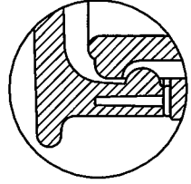
カバー簡易ロック機能部図 2/1
