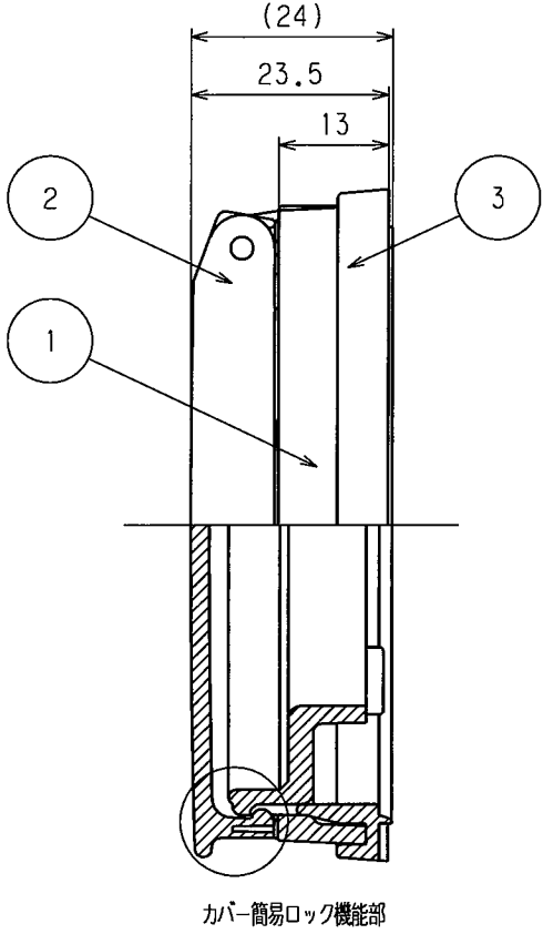
カバー簡易ロック機能部
