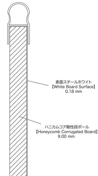
ホワイトボード (断面図) 【White Board - Cross Section】
