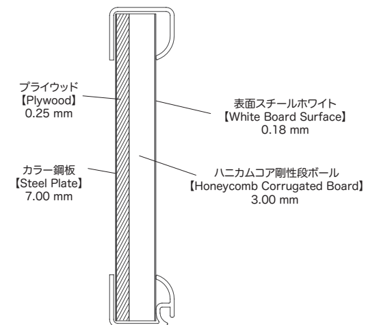
ホワイトボード (断面図) 【White Board - Cross Section】
