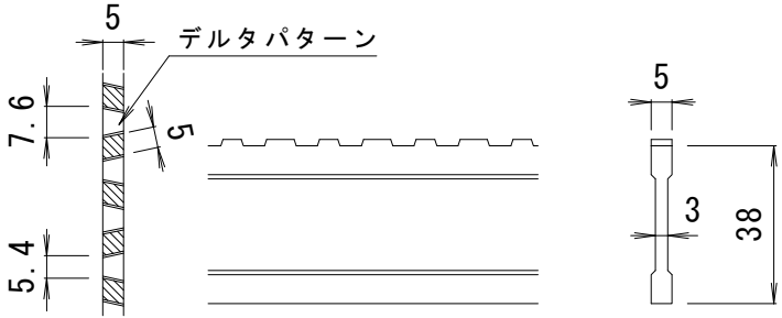
D I - 38 バー形状詳細 S = 1 : 2
