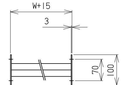
アングル支手 S (1:5)
