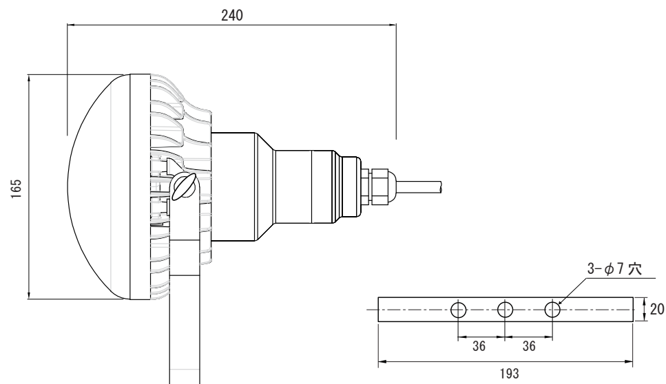
取付穴寸法
