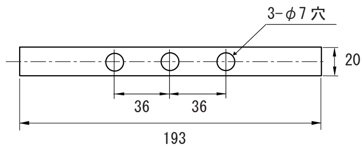
取付穴寸法
