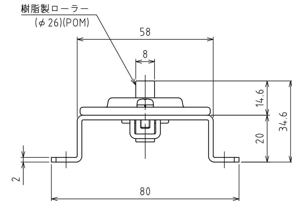
A矢視図
