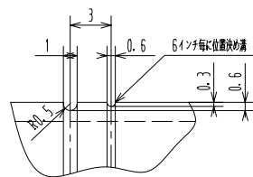
"Z" 詳細
