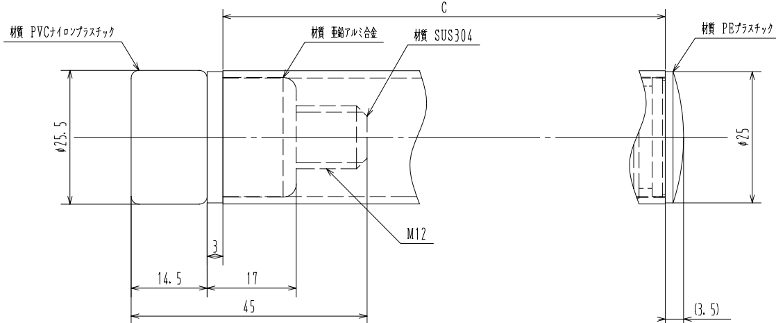
アジャスター、キャップ取付詳細
