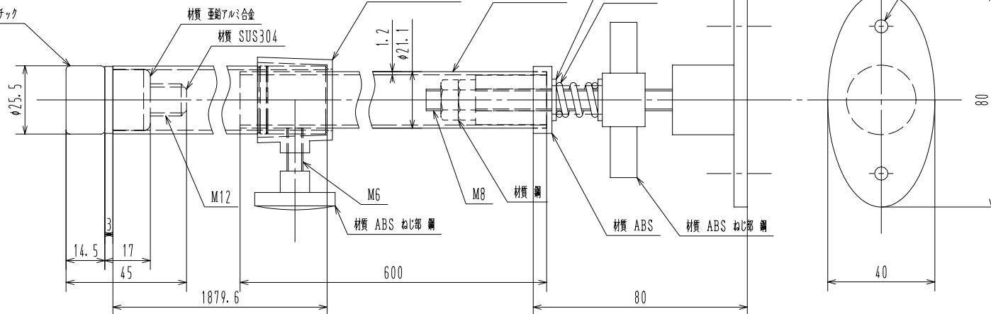
組立図
