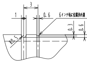
"Z" 詳細
