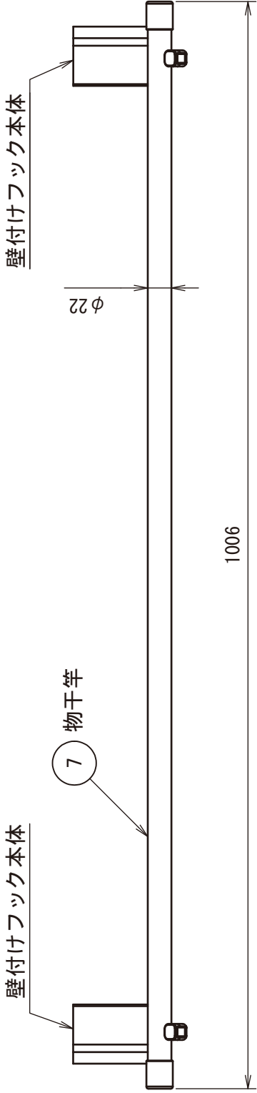
＜物干竿を掛けた状態図＞
