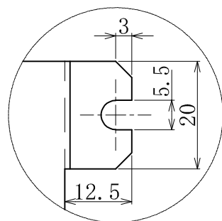
C部詳細
