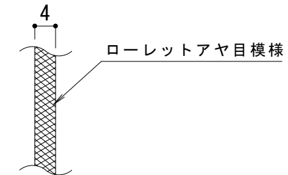
メインバー表面 S = 1 : 1
