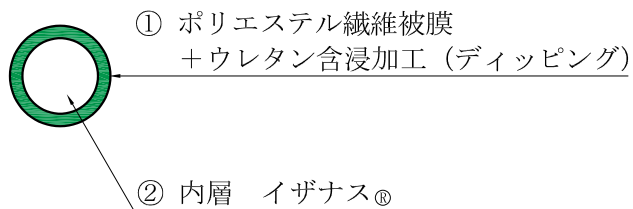
ロープ断面図
