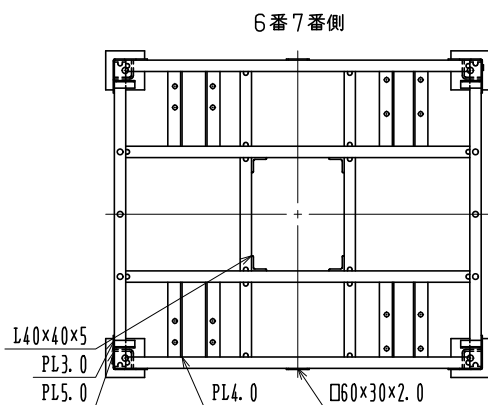
2番3番側 金網を除いたベース上面詳細
